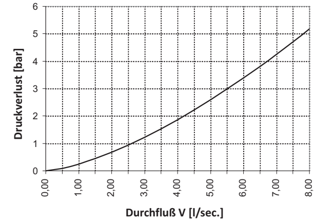
Druckverlust Nutzwasser:
