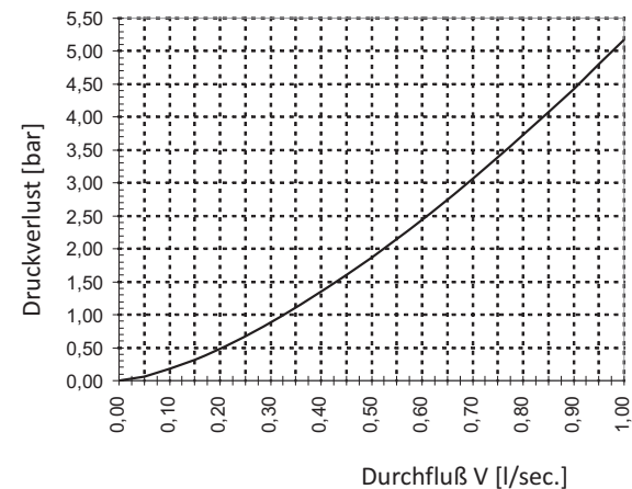
Druckverlust Nutzwasser:
