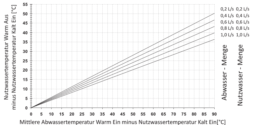
Temperaturkennlinien:
