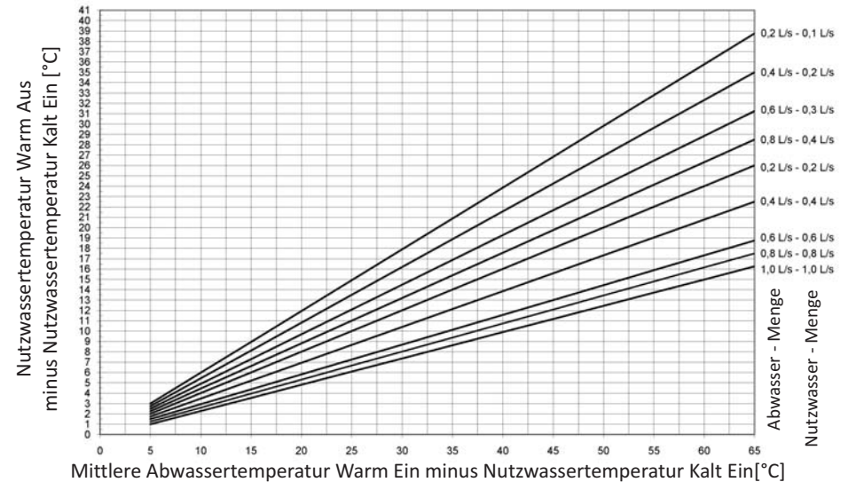
Temperaturkennlinien:
