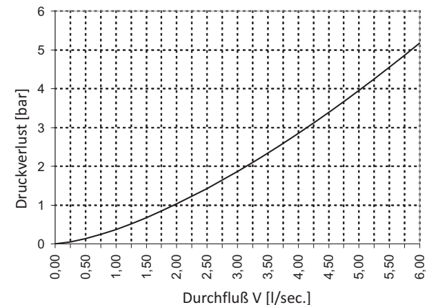
Druckverlust Nutzwasser:
