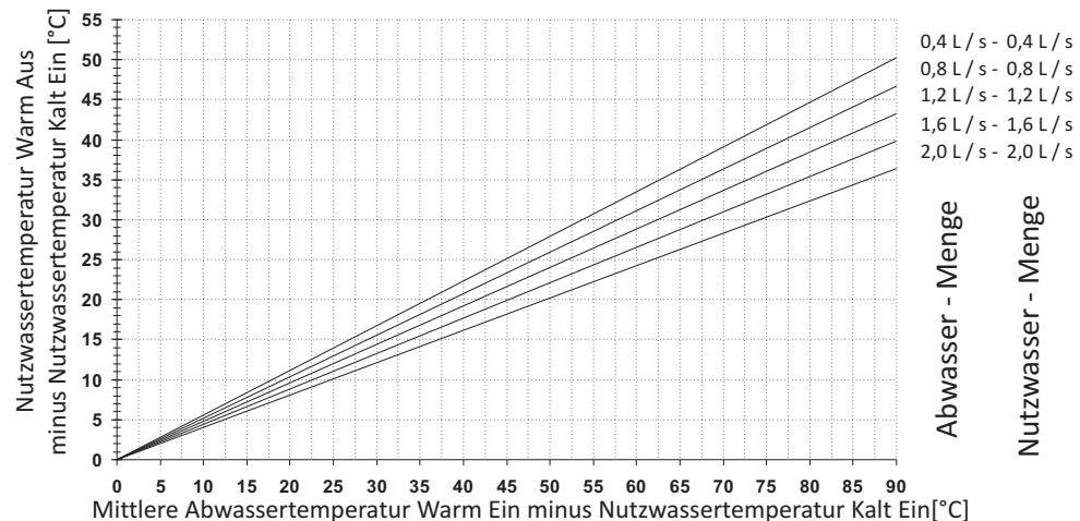
Temperaturkennlinien:
