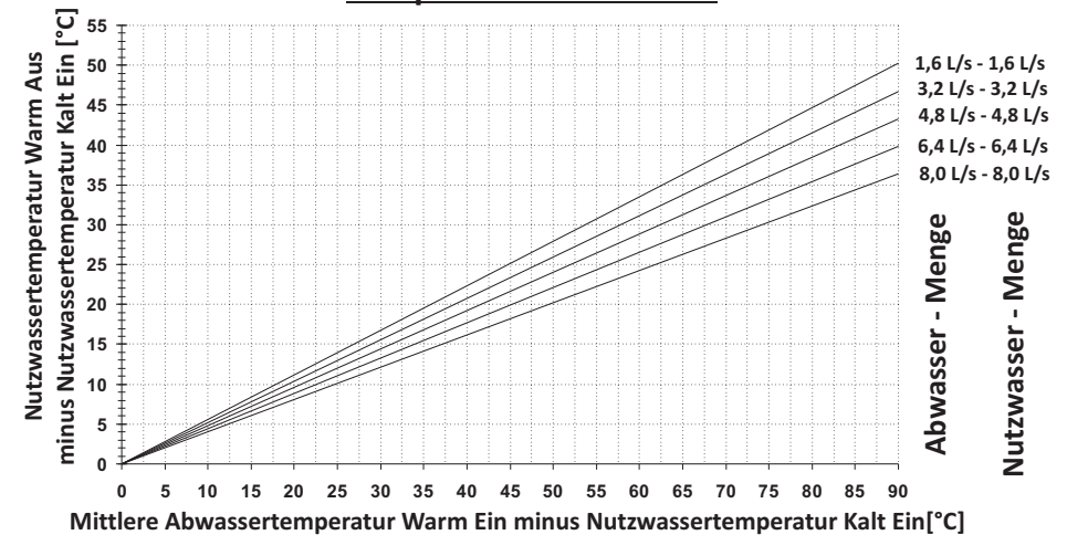
Temperaturkennlinien:
