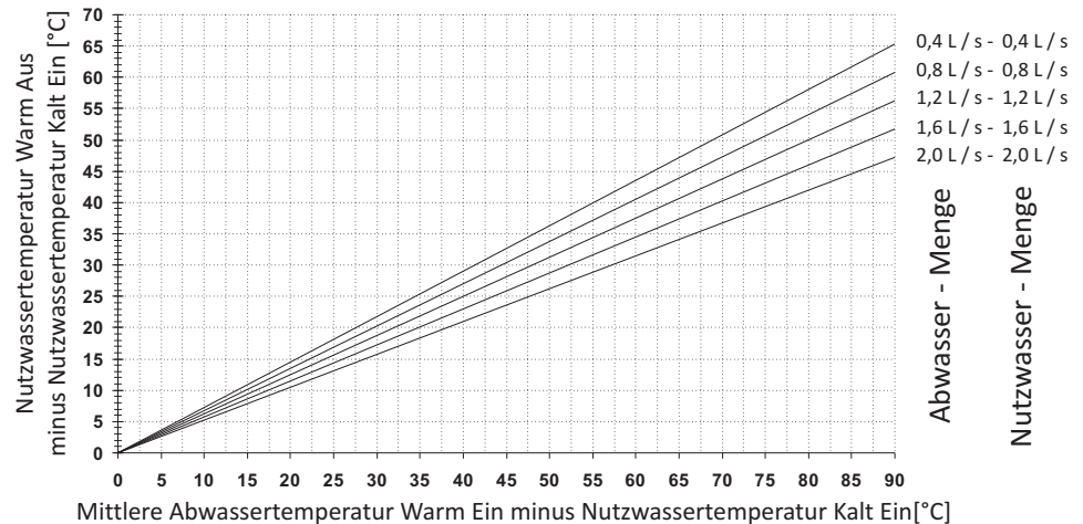
Temperaturkennlinien:
