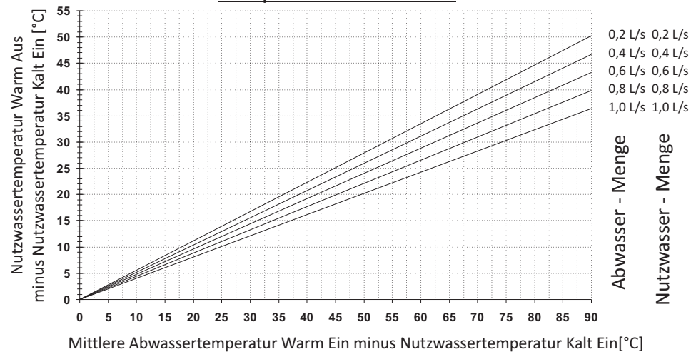
Temperaturkennlinien:
