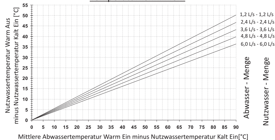
Temperaturkennlinien:
