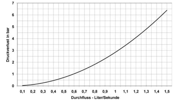
Druckverlust Nutzwasser:
