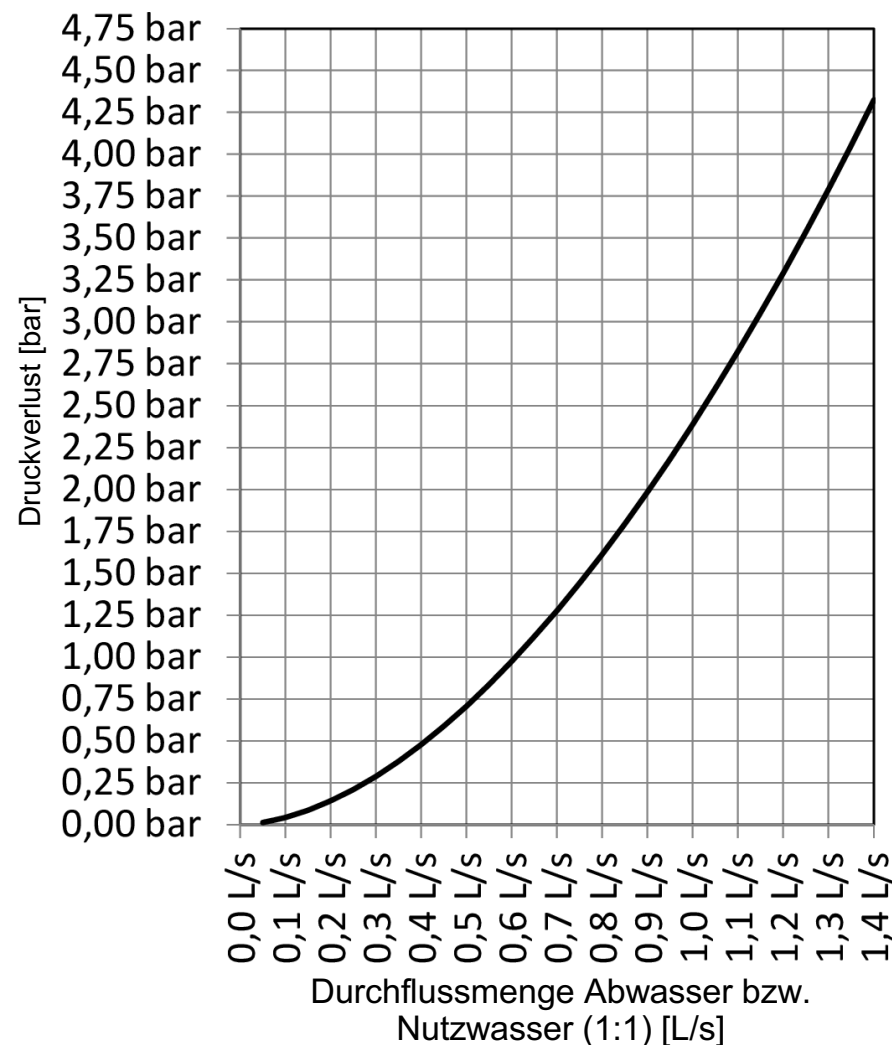
Nutzwasser-Druckverlust
