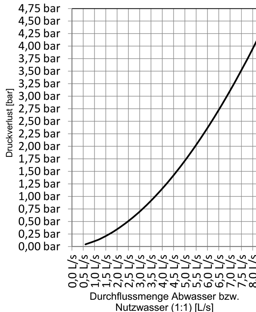
Nutzwasser-Druckverlust
